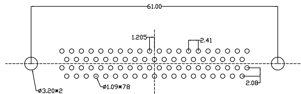
P.C.B LAYOUT
