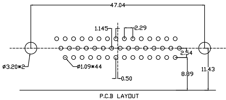
P.C.B LAYOUT
