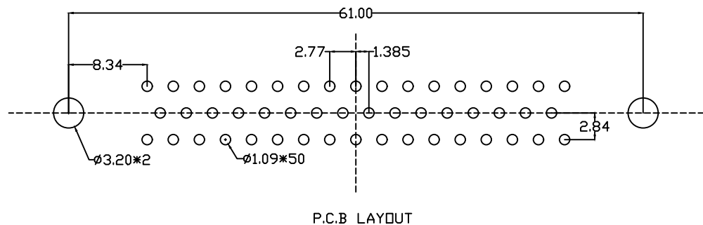
P.C.B LAYOUT
